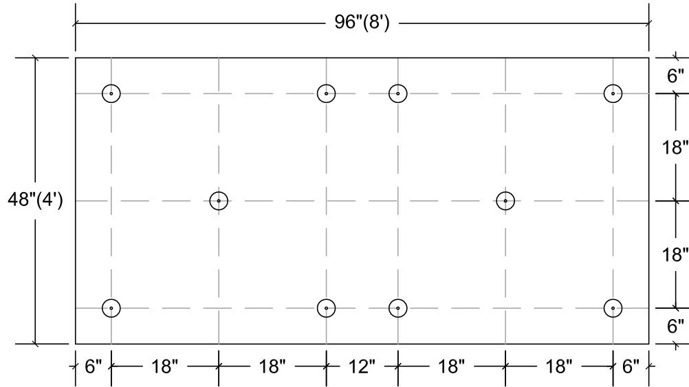
10 FASTENERS PER 4 X 8
