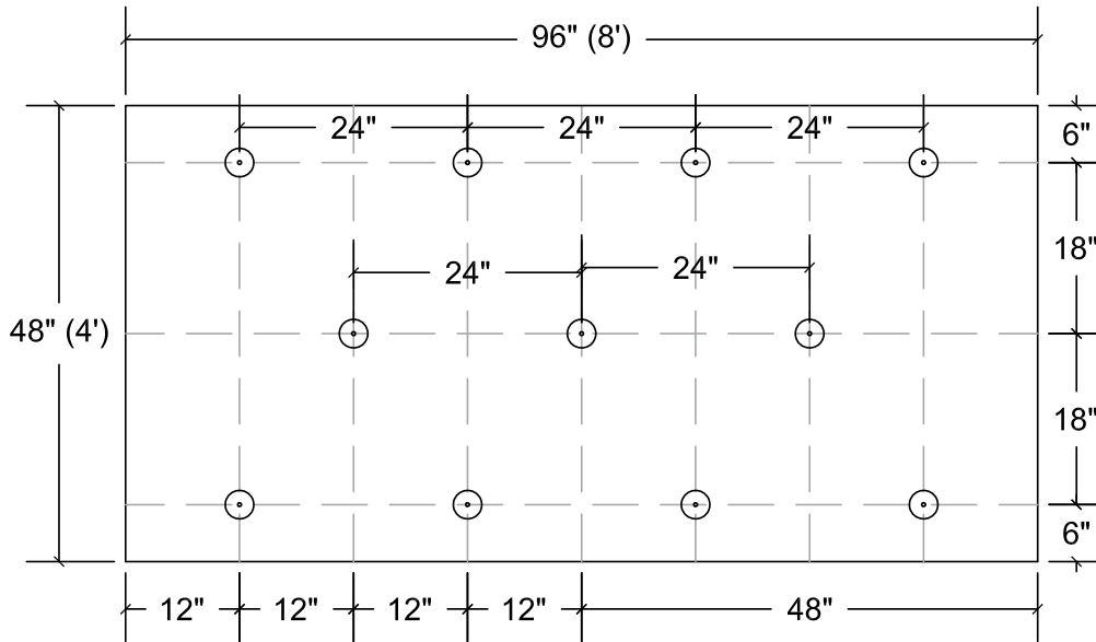
11 FASTENERS PER 4 X 8
